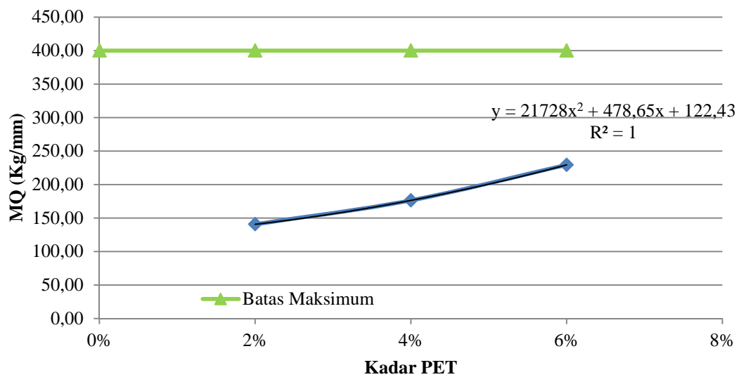
Gambar 6 Hubungan kadar PET dalam campuran aspal pori dengan MQ
