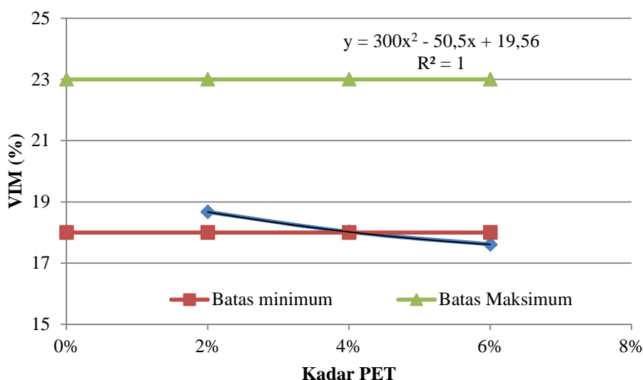
Gambar 4 Hubungan kadar PET dalam campuran aspal pori dengan VIM
