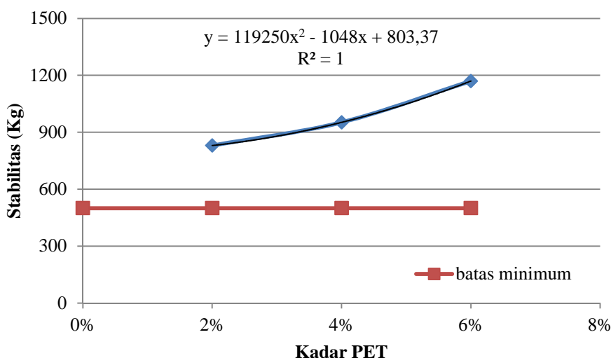
Gambar 3 Hubungan kadar PET dalam campuran aspal pori dengan stabilitas
