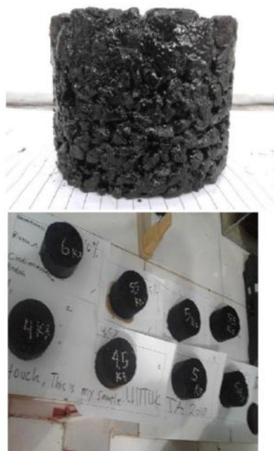
Gambar 2. Sampel pengujian Marshal
