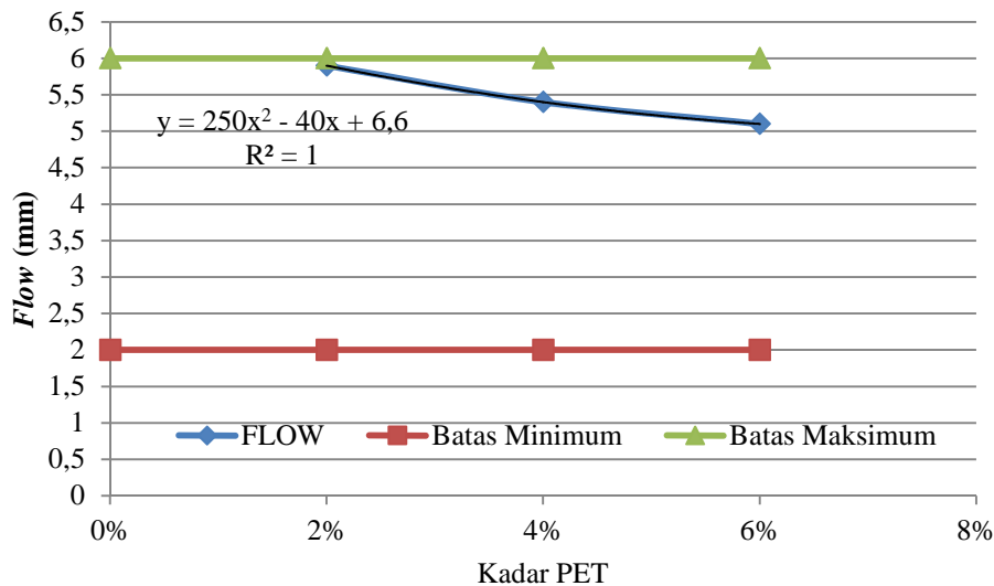
Gambar 5 Hubungan kadar PET dalam campuran aspal pori dengan Flow
