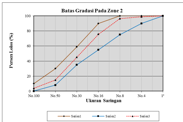
Gambar 2. Grafik Gradasi agregat halus (pasir) pada quarry PT. Sari Wagon
