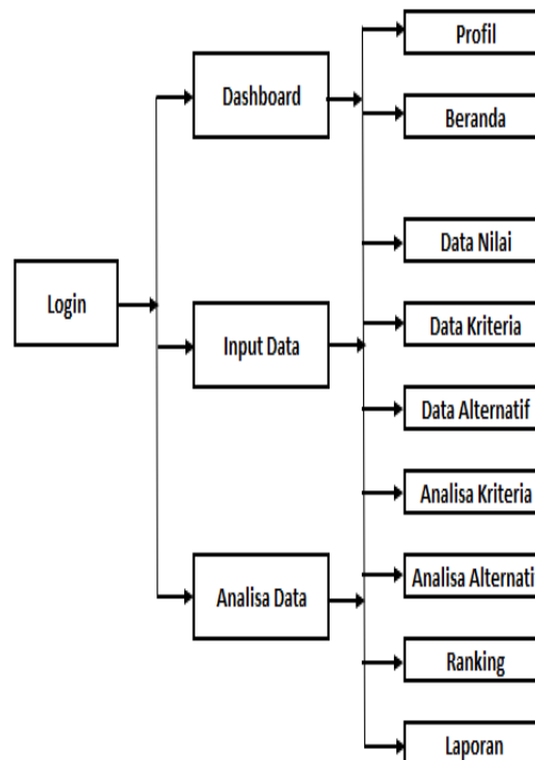
Gambar 3. Struktur Menu
